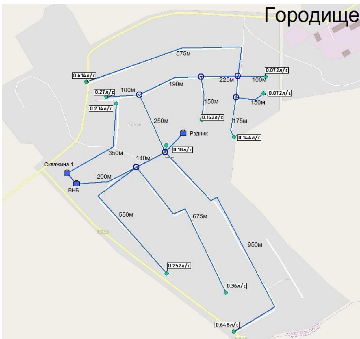
Рисунок 1.1.3.3 - Зона централизованного водоснабжения н.п. Городище
