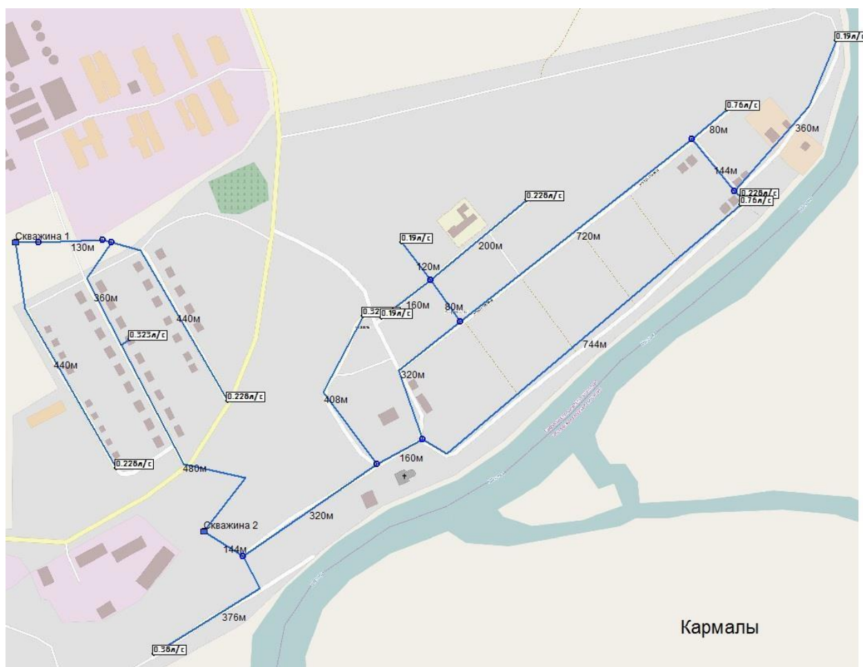
Рисунок 1.1.3.1 - Зона централизованного водоснабжения с.Кармалы
